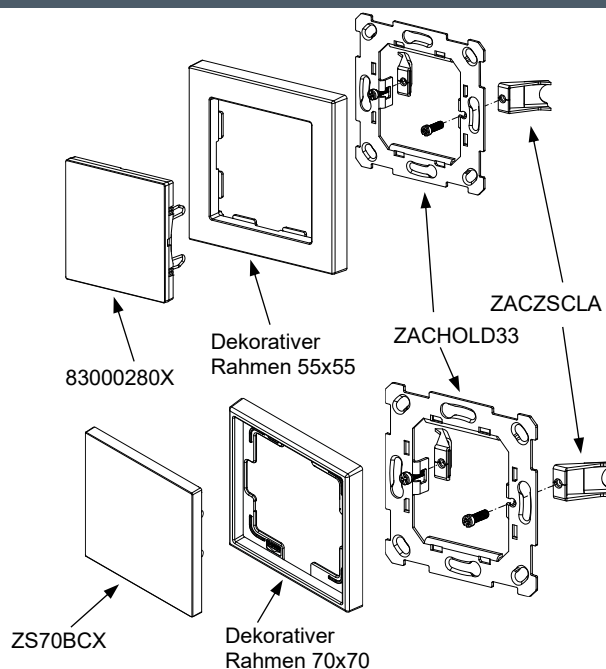
Abbildung 1: Blindabdeckung.
